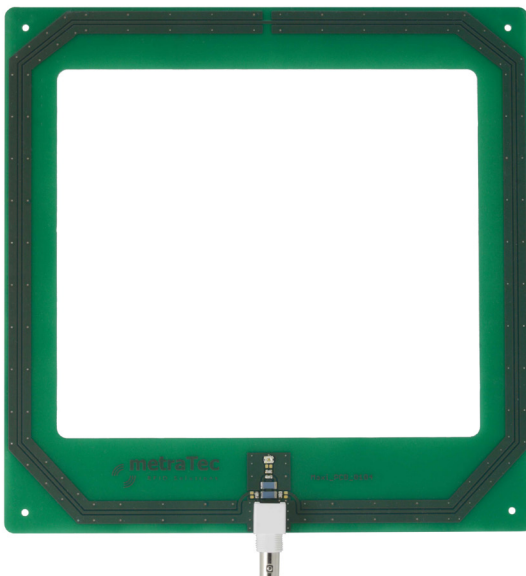
MaxiPCB Antenne Art.-No.: 2200 0027
