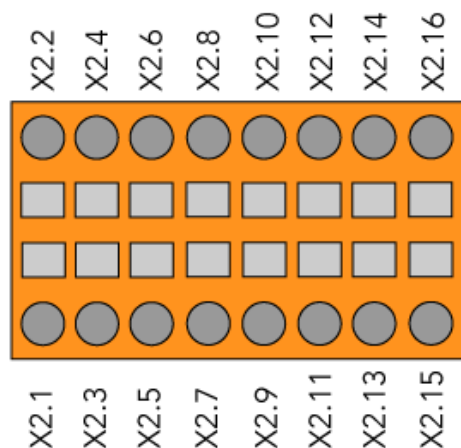
Abb. 3: Steckerbelegung PulsarMX
